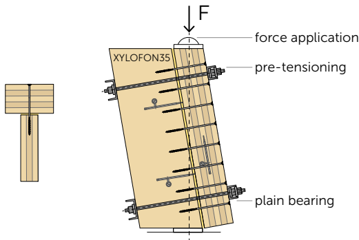
TEST [ T-X ] (CLT - XYLOFON35 - CLT)
